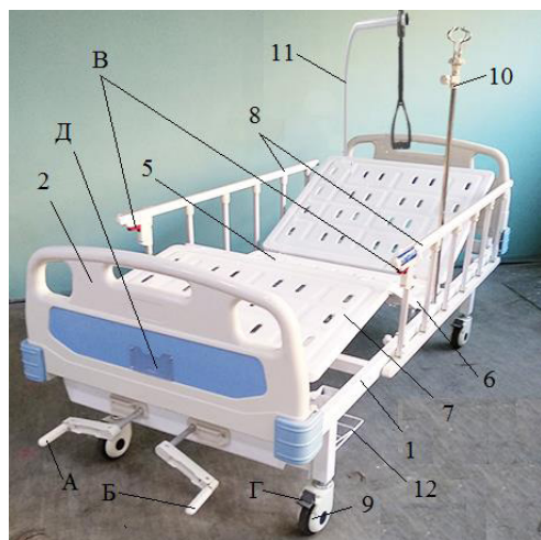
Рис.2. Основные части кровати Barry MB2pp (на рисунке матрас не показан) и органы ее управления.
