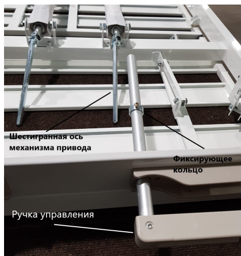
Рис. 7. Установка ручки управления привода
