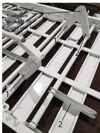
Рис. 8 – Схем установки рычагов наклона
